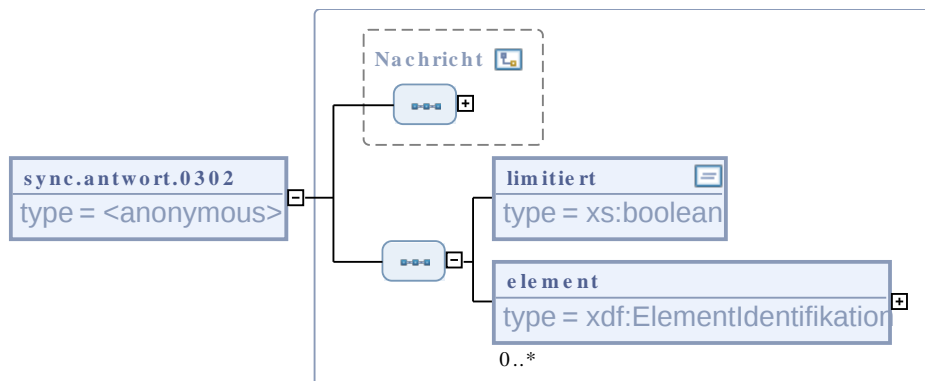
Abbildung III.1.10. sync.antwort.0302
