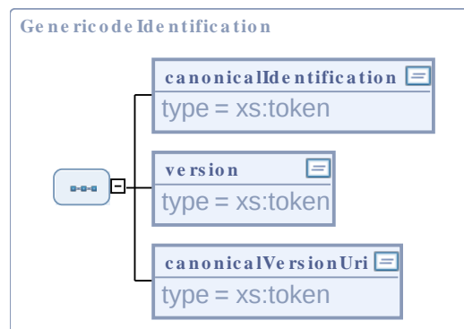
Abbildung II.3.10. GenericodeIdentification
