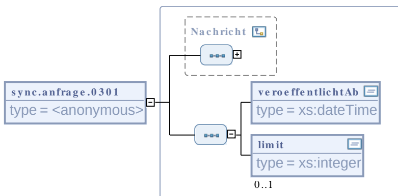
Abbildung III.1.9. sync.anfrage.0301
