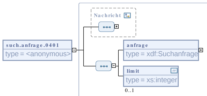
Abbildung III.1.12. such.anfrage.0401
