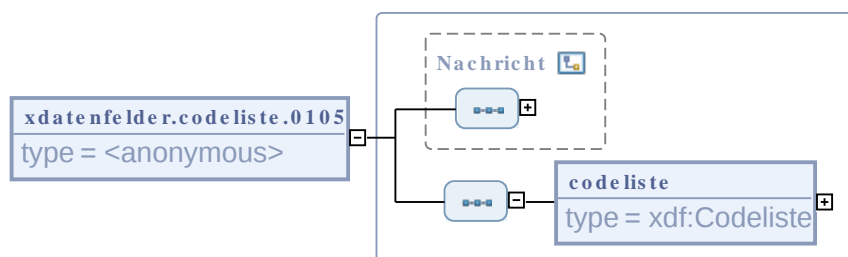
Abbildung III.1.5. xdatenfelder.codeliste.0105
