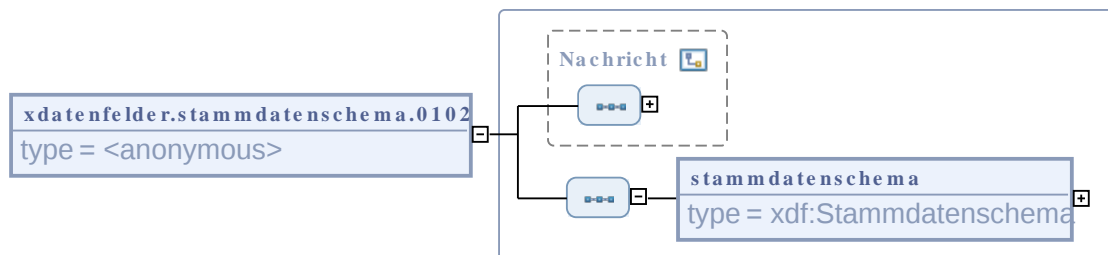
Abbildung III.1.2. xdatenfelder.stammdatenschema.0102
