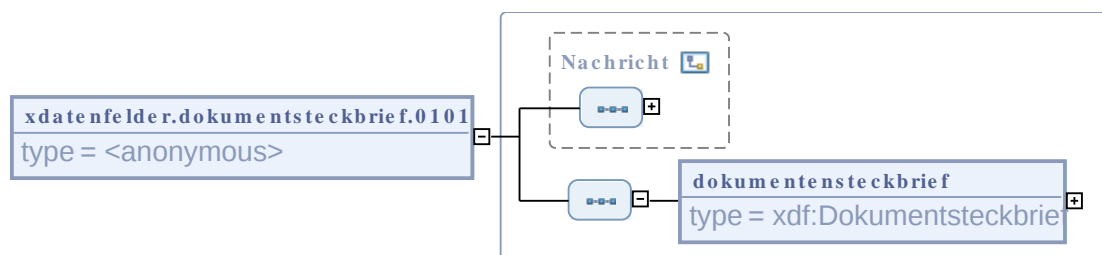
Abbildung III.1.1. xdatenfelder.dokumentsteckbrief.0101
