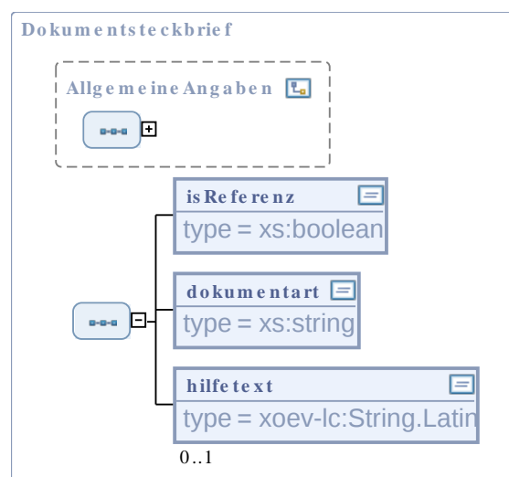
Abbildung II.3.6. Dokumentsteckbrief
