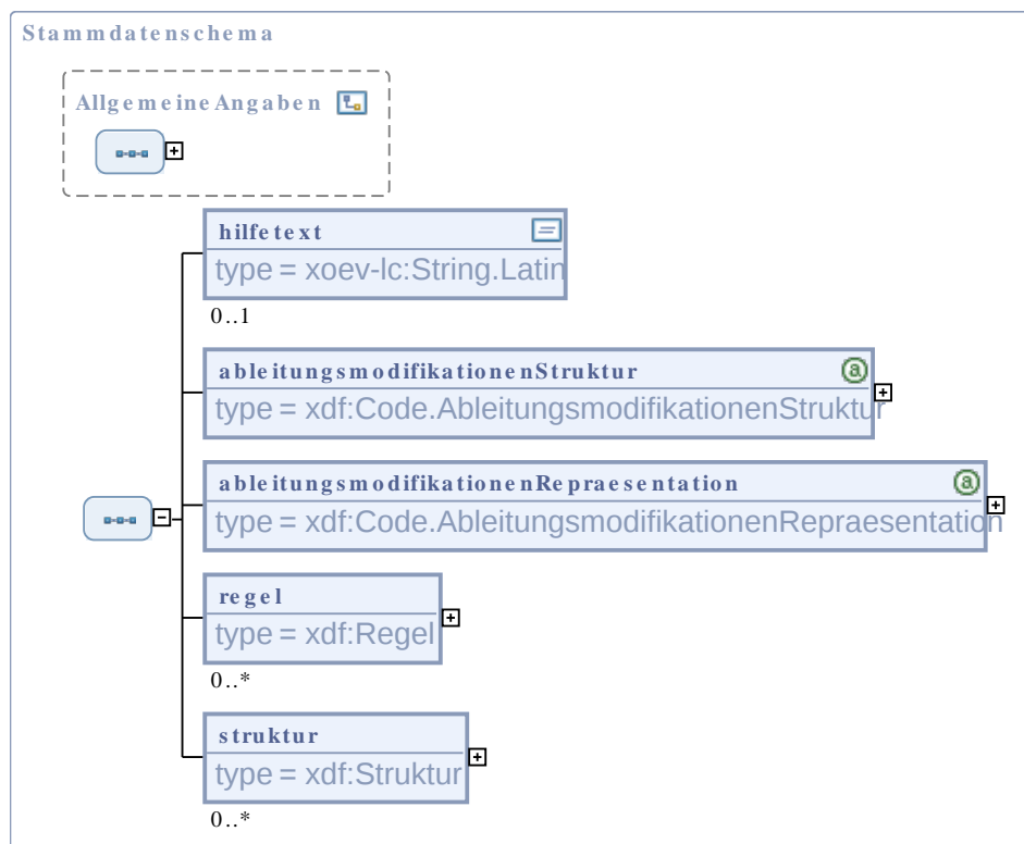
Abbildung II.3.15. Stammdatenschema
