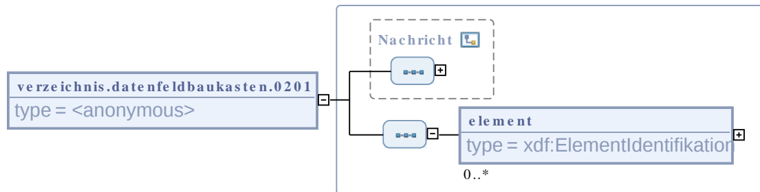
Abbildung III.1.6. verzeichnis.datenfeldbaukasten.0201
