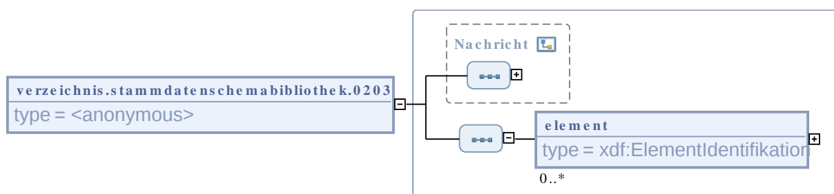
Abbildung III.1.8. verzeichnis.stammdatenschemabibliothek.0203
