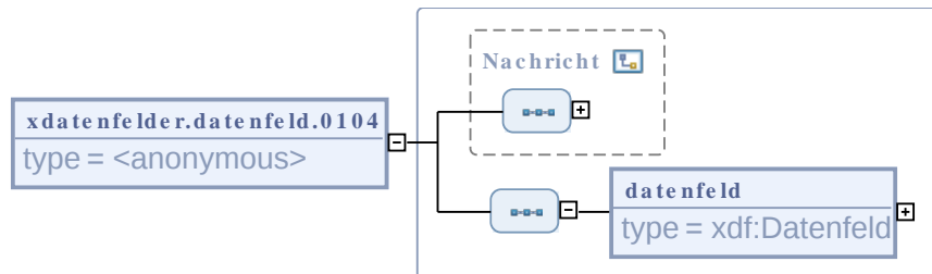
Abbildung III.1.4. xdatenfelder.datenfeld.0104
