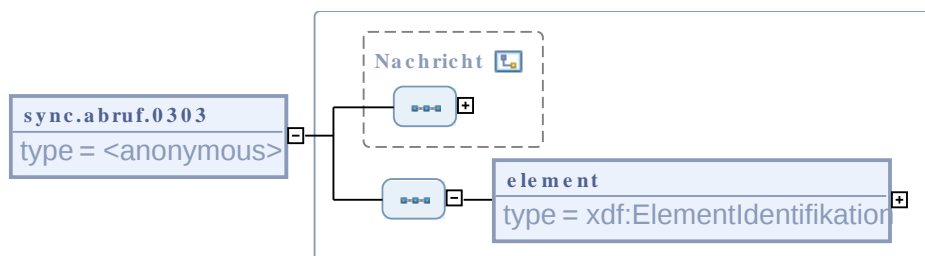
Abbildung III.1.11. sync.abruf.0303
