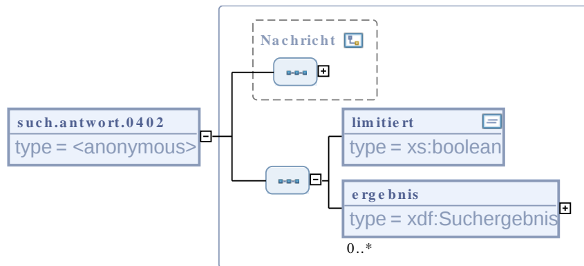
Abbildung III.1.13. such.antwort.0402
