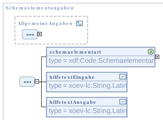
Abbildung II.3.14. Schemaelementangaben
