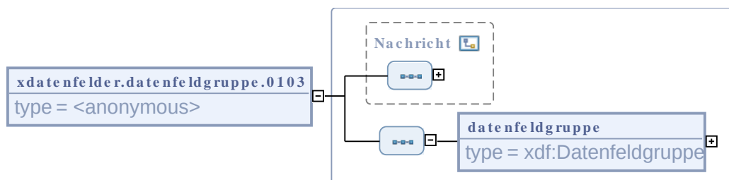
Abbildung III.1.3. xdatenfelder.datenfeldgruppe.0103
