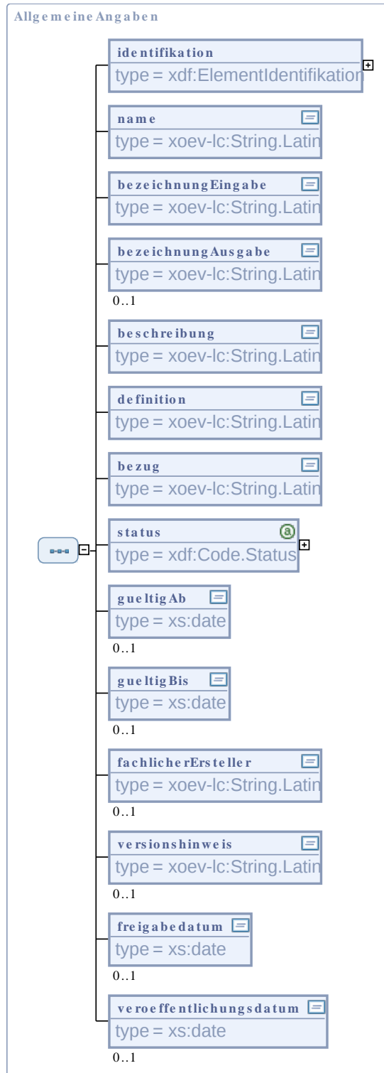
Abbildung II.3.1. AllgemeineAngaben
