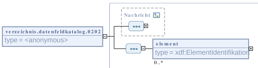
Abbildung III.1.7. verzeichnis.datenfeldkatalog.0202
