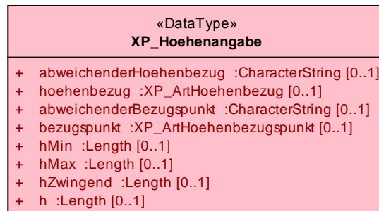
Abbildung 7: XPlanung Datenstruktur zur Spezifikation einer Höhenangabe (UML-Modell)
